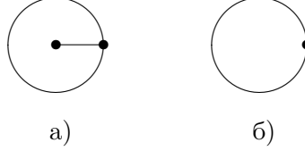
Рис. 2. Клеточные разбиения диска D^2 .
