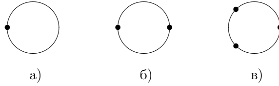
Рис. 1. Псевдосимплициально клеточные разбиения окружности.
