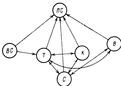
Рис. 2.1. Пути перехода к иным калибровкам матрицы
