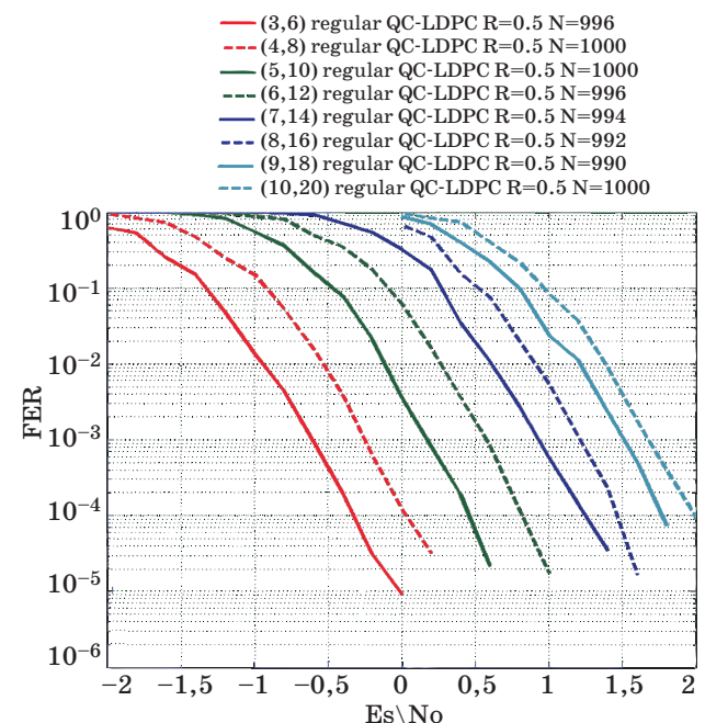
■ Рис. 3. Зависимость вероятности ошибки на блок (FER) от отношения сигнал/шум на кодированный бит ( E_s/N_0 ) для регулярных квазициклических МПП-кодов при различном числе слоев l
